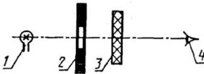
1 — источник света, 2 — непрозрачный экран с отверстием, 3 — образец, 4 — глаз контролера. Черт. 1
